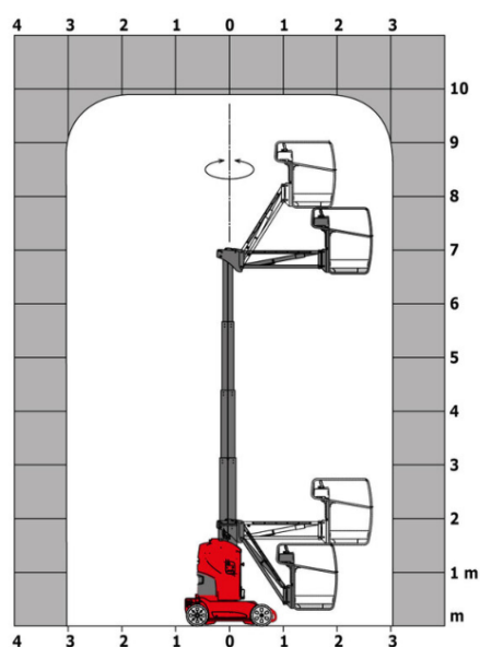
Діаграма для підйомної платформи
