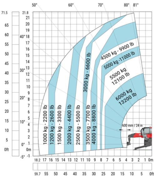
Машина на опущених стабілізаторах з вилами (CAF)
