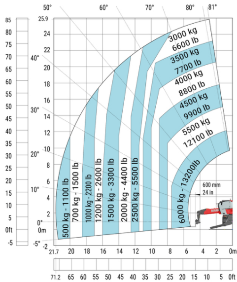
Машина на опущених стабілізаторах з вилами (CAF)
