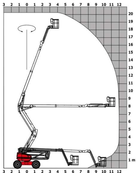
Діаграма навантаження
