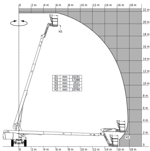
Діаграма для підйомної платформи
