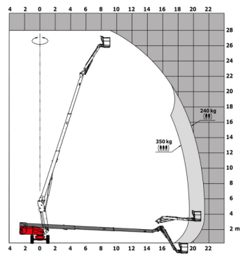
Діаграма для підйомної платформи
