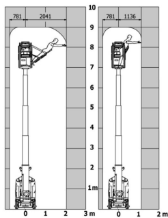
Діаграма для підйомної платформи
