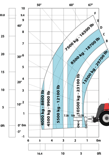
Машина на шинах з 3-гаким гуськом 13 500 кг
