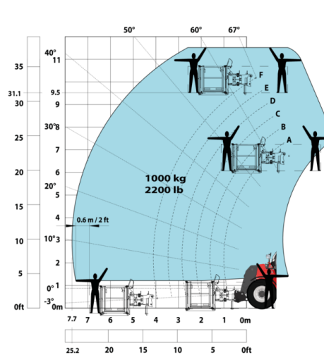
Машина на шинах з платформою
