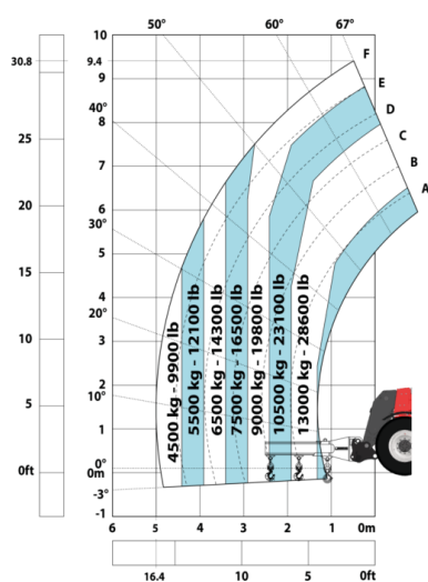
Машина на шинах з 3-гаквим гуськом 16 000 кг
