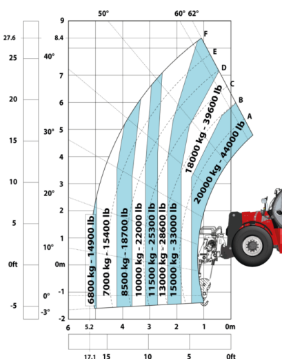
Машина на шинах з лебідкою 20 000 кг
