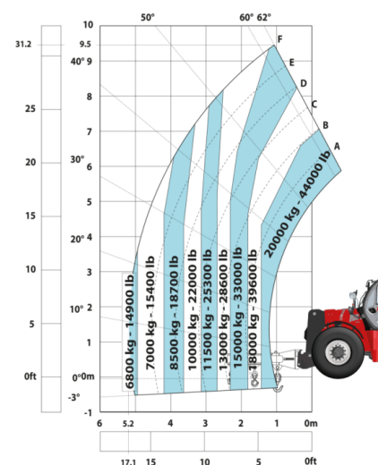
Машина на шинах з 3-гаквим гуськом 20 000 кг
