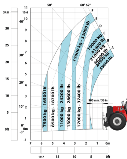
Машина на шинах з лебідкою 25 000 кг
