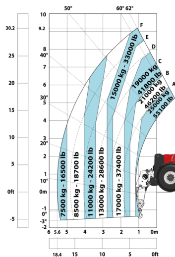
Машина на шинах з лебідкою 25 000 кг
