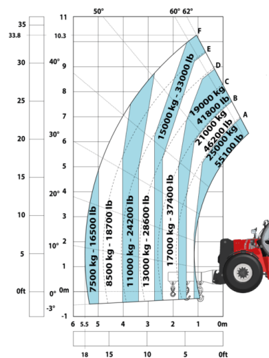
Машина на шинах з 3-гаківим гуськом 25 000 кг
