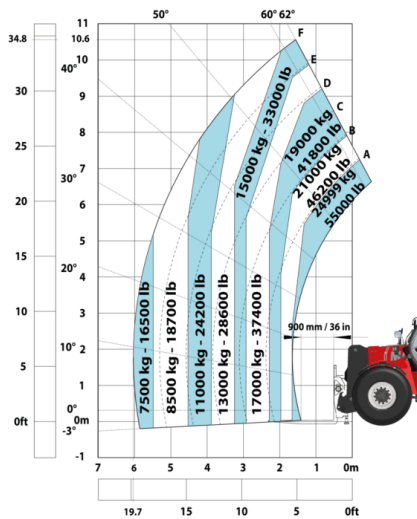
Машина на шинах з лебідкою 25 000 кг
