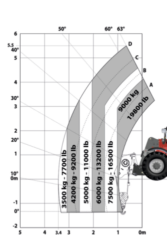
Машина на шинах з лебідкою 9 000 кг
