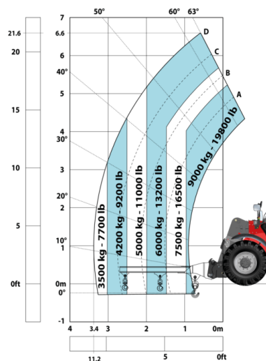
Машина на шинах з 3-гачовим гуськом 9 000 кг
