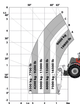
Машина на шинах з лебідкою 9 000 кг
