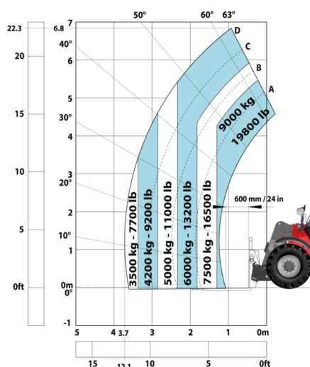
Машина на шинах з 3-гачим гуськом 9 000 кг
