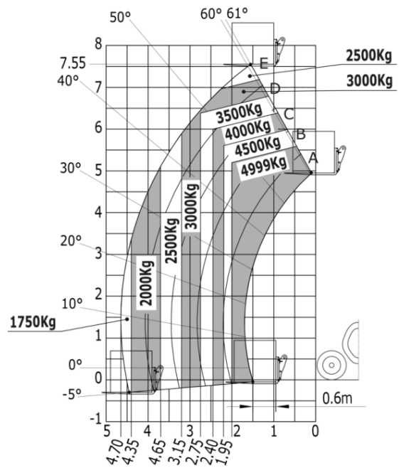
Машина на шинах з вилами · центр ваги 600 мм
