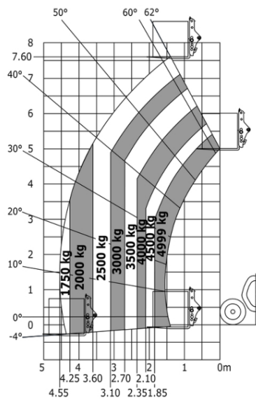
Машина на шинах з вилами
