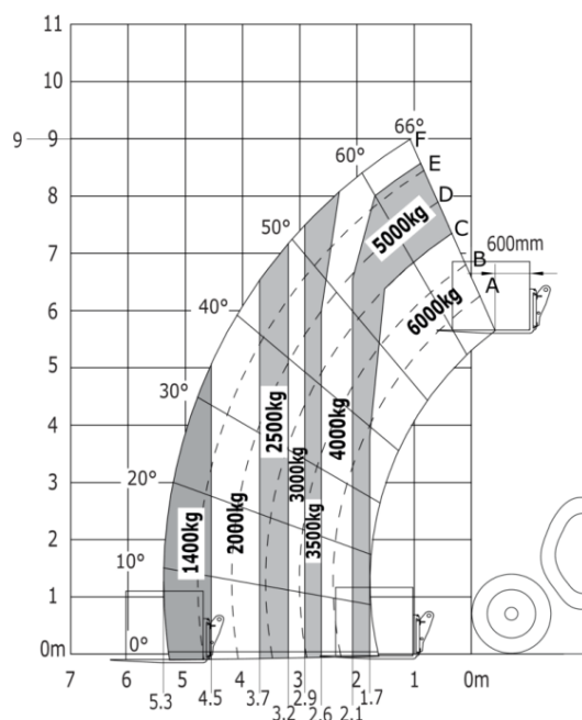
Машина на шинах з вилами - центр ваги 600 мм
