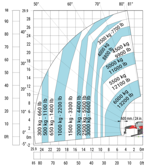
Машина на опущених стабілізаторах з вилами (CAF)
