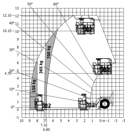
Машина на опущених стабілізаторах з тунельною платформою (Metric)
