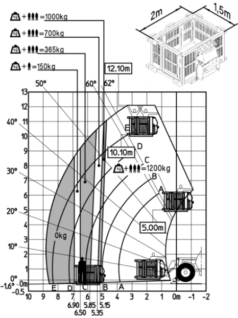
Машина на опущених стабілізаторах, підземні роботи platform (Metric)
