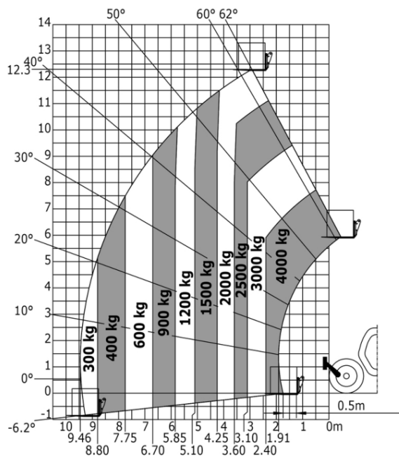
Машина на шинах з вилами · з механізмом вирівнювання
