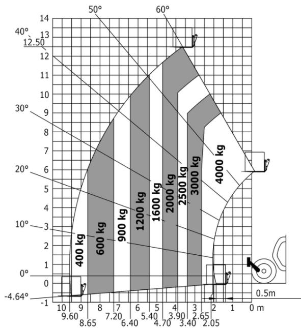
Машина на шинах з вилами · з механізмом вирівнювання
