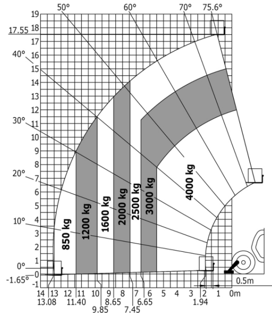
Машина на опущених стабілізаторах з вилами
